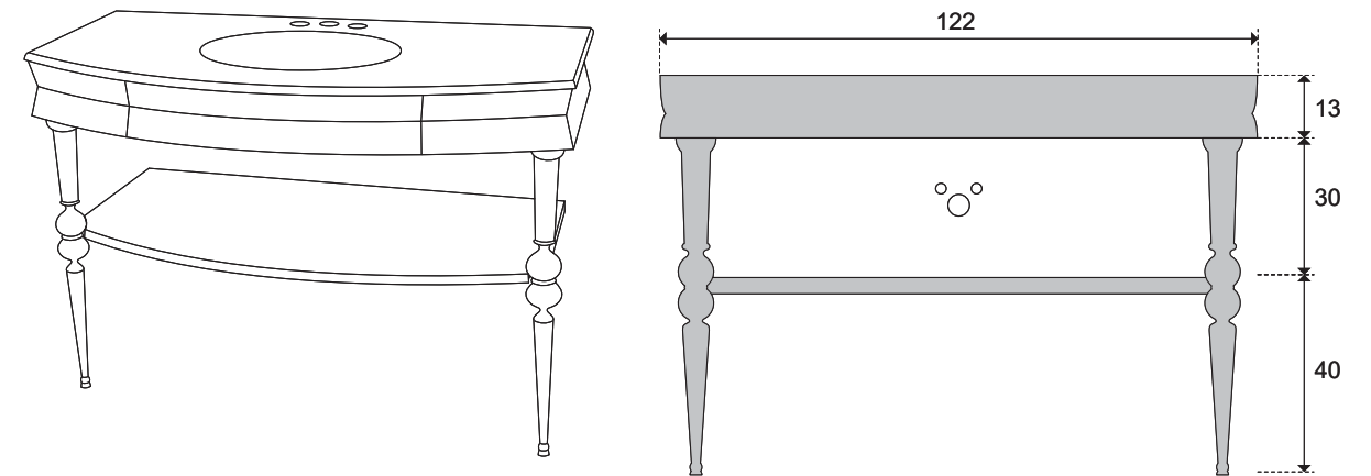
FASHION FH-M124G BASE P/LAVABO SINGOLO CON RIPIANO SOTTOSTANTE IN LEGNO E GAMBE METALLICHE BASE FOR ONE WASHBASIN WITH WOODEN SHELF AND METAL LEGS ТУМБА ПОД ОДНУ РАКОВИНУ С ДЕРЕВЯННОЙ ПОЛКОЙ И МЕТАЛЛИЧЕСКИМИ НОЖКАМИ
